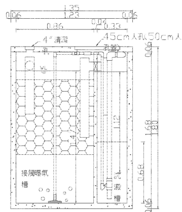
處理設施B-B側視圖
