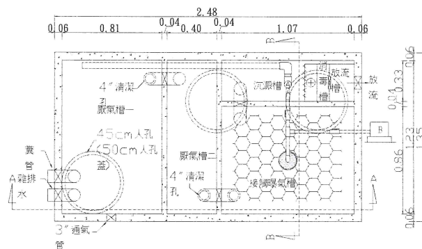
處理設施俯視圖 單位 m
