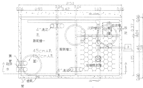
處理設施俯視圖 單位:m
