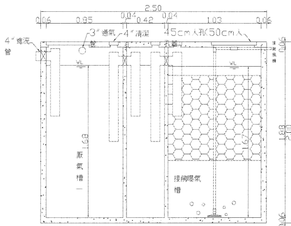
處理設施A-A剖面圖 單位:m
