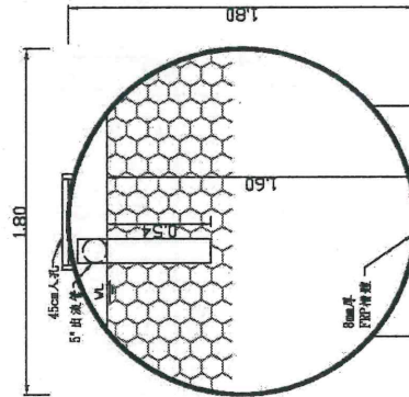
厭氣濾床槽B-B剖面圖 單位：mm 比例：1/30
