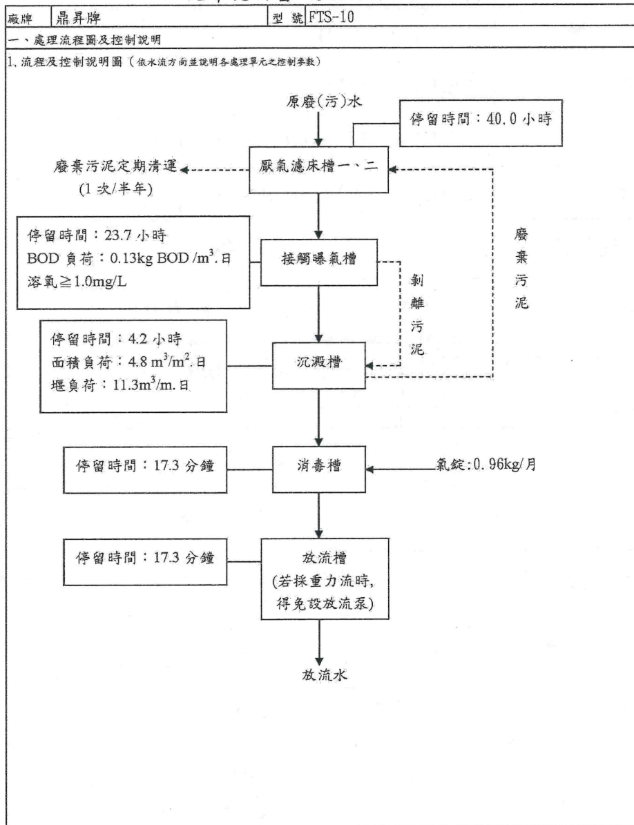
設計說明書—處理流程圖及設施概要(1)
