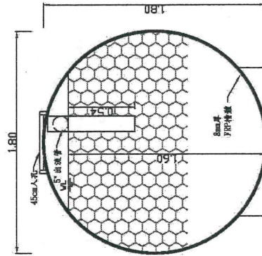
厭氣濾床槽C-C剖面圖 單位：mm 比例：1/30
