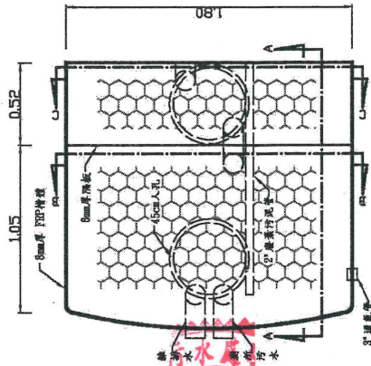
厭氣濾床槽俯視圖 單位：mm 比例：1/30
