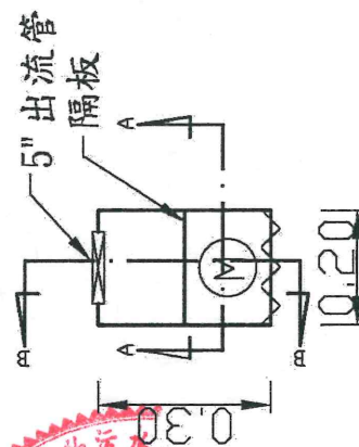
消毒槽俯視圖 單位m 比例1/10
