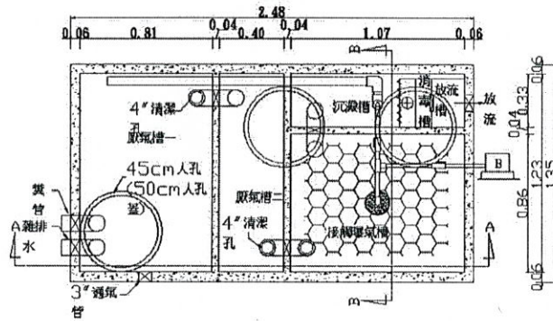
處理設施俯視圖 單位m
