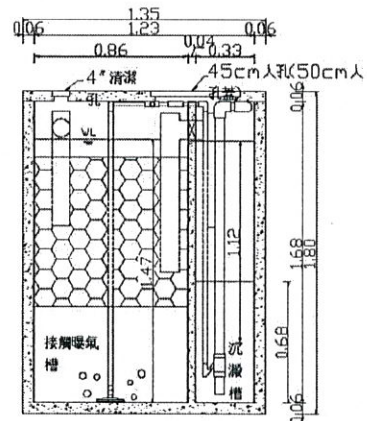
處理設施B-B側視圖
