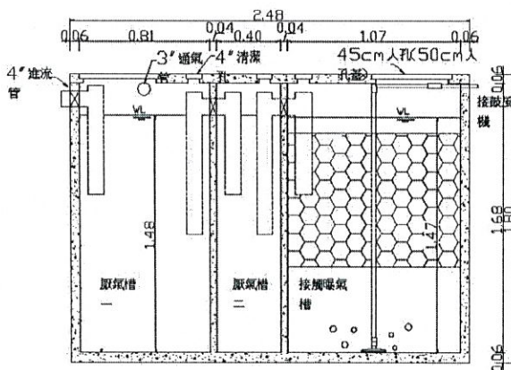
處理設施A-A剖面圖 單位m
